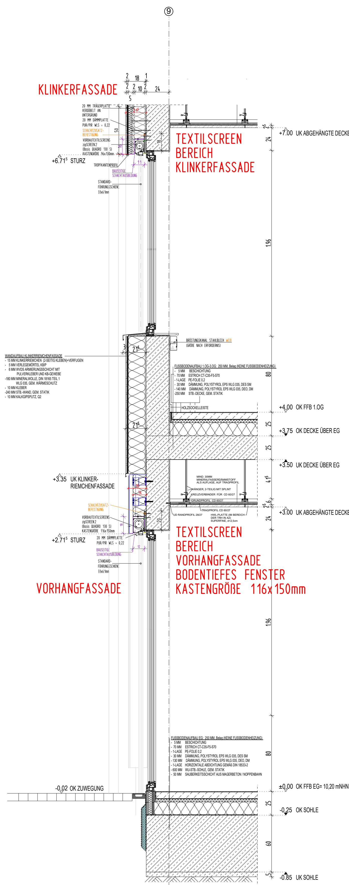
FASSADENSCHNITT 2 TEILSCHNITT
